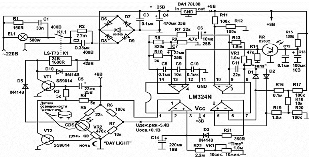
Рисунок 3. Схема датчика движения
