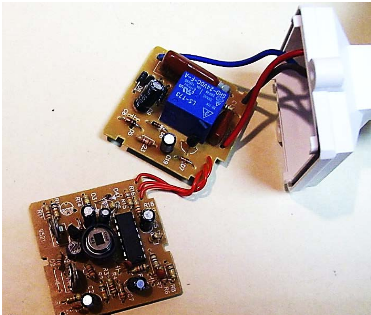
Рисунок 1. Вид со стороны детали
