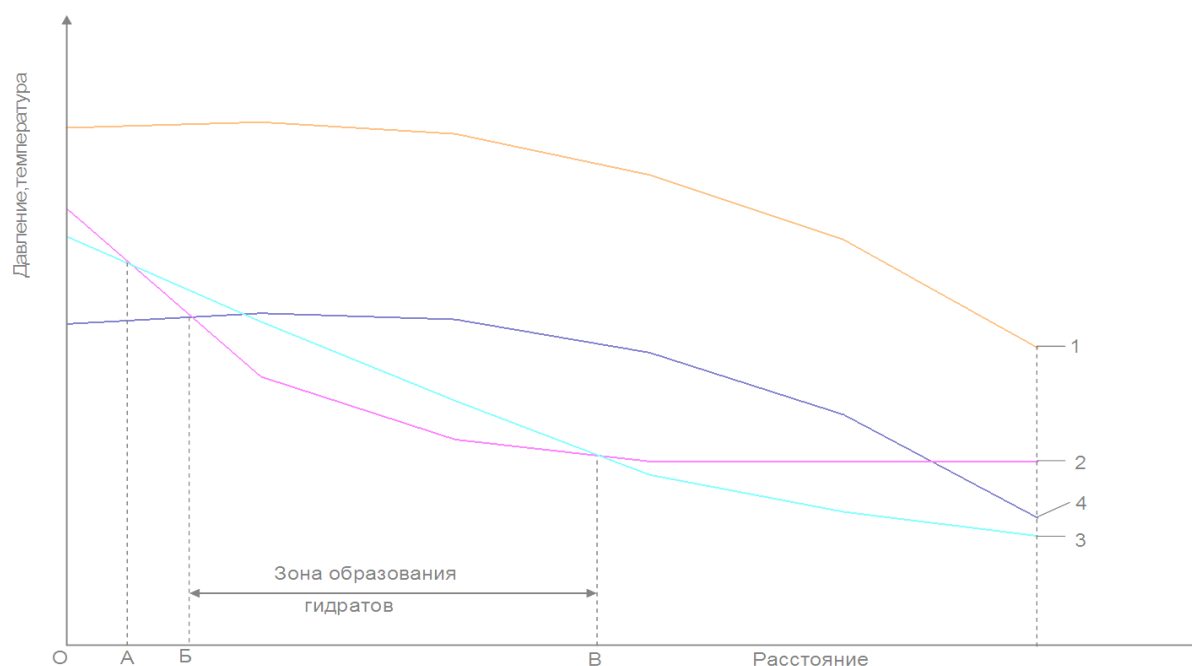
Рис. 2. Изменение условий образования гидратов в шлейфе скважины, точка 1 – изменение давления по длине шлейфа, 2 – изменения температуры газа по длине шлейфа; 3 – изменение точки по длине шлейфа, 4 – изменение температуры образования гидратов при различных давлениях
