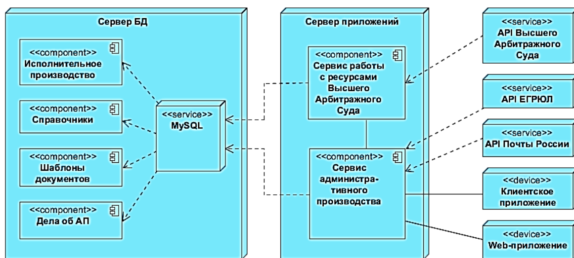
Рис. 2. Диаграмма развертывания системы
