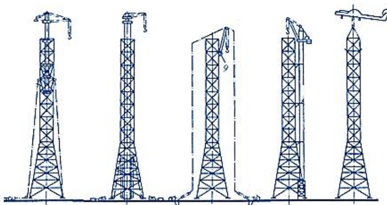
Рис. 1. Различные способы монтажа башни при наращивании
