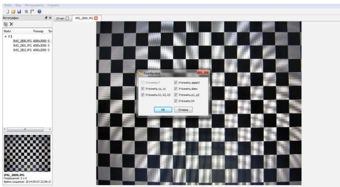
Рис. 2. Выбор параметров калибровки в Agisoft Lens
