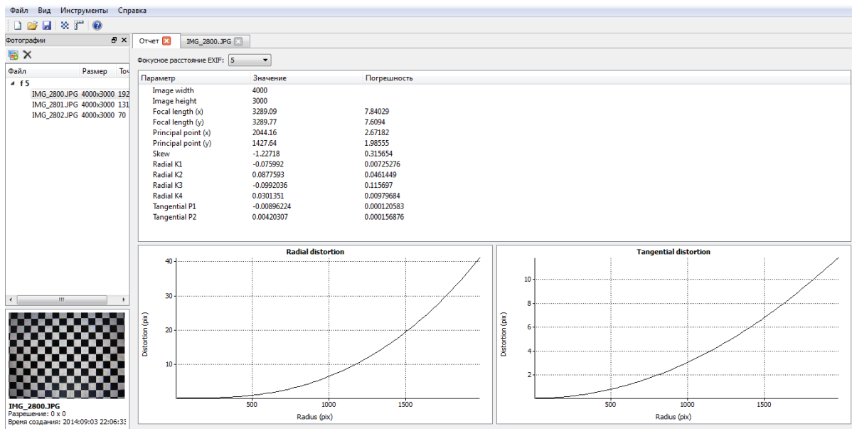
Рис. 3. Результат калибровки цифровой фотокамеры
