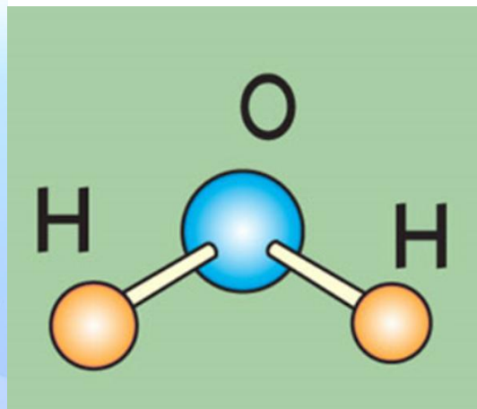
Молекула воды (H 2 O)
