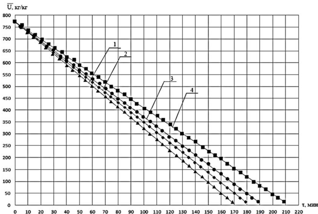
Рис. 2. График процесса сушки измельченной цветной капусты инфракрасным излучением высотой слоя 10 мм и эквивалентным диаметром 1 мм (кривая 1) и 2 мм (кривая 2) при плотности теплового потока 3,9 \text{ кВт/м}^2 , эквивалентным диаметром 1 мм (кривая 3) и 2 мм (кривая 4) при плотности теплового потока 3,55 \text{ кВт/м}^2
