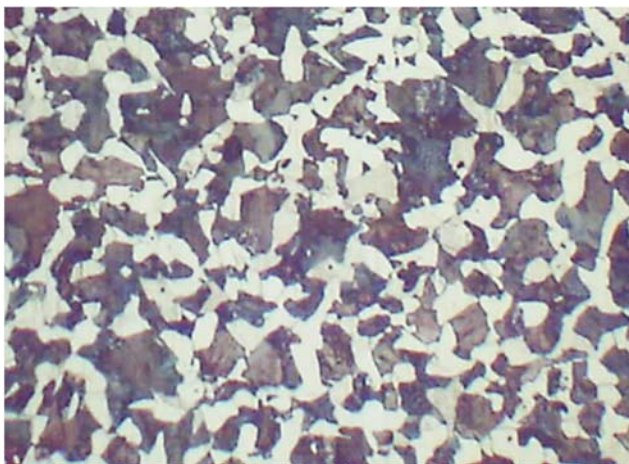
Рис. 8. Микроструктура зубьев шестерен редуктора мотокультиватора «Крот»
