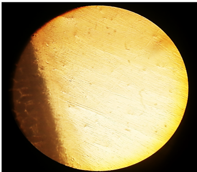
Рис. 5. Азотированный слой в образце из сплава 5 ВМЦ, прошедшего насыщение при 550^{\circ}\text{C} в течение 8 часов (x150)
