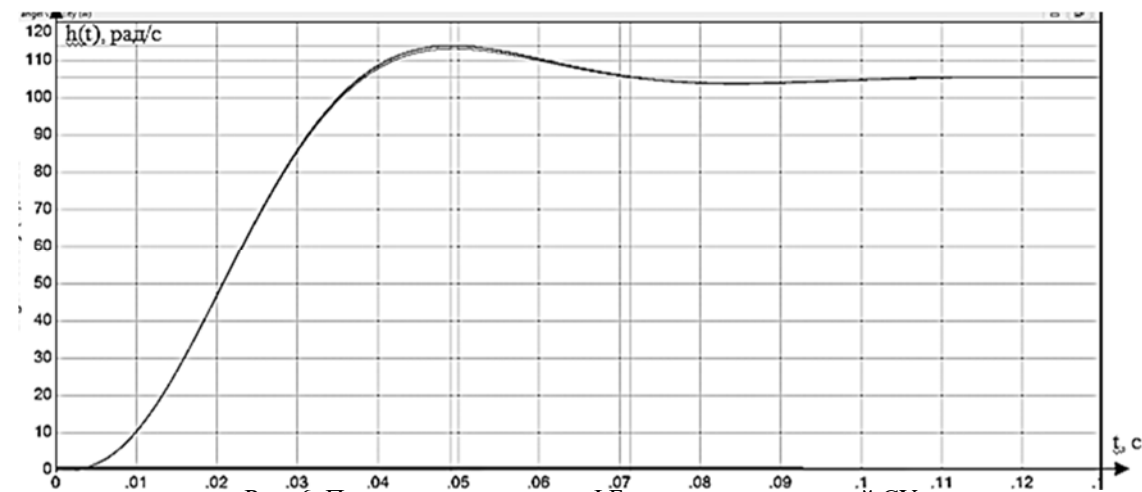
Рис. 6. Переходные процессы ФБ и скорректированной СУ
