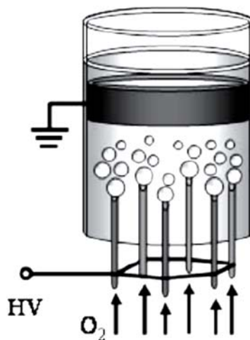
Рис. 1. Реактор для очистки воды [1]
