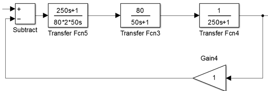
Рис. 2. Структурная схема замкнутой системы температуры в климатической камере
