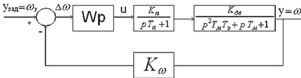
Рис. 2. Структурная схема синтезируемой замкнутой системы
