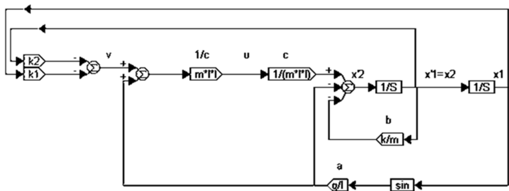
Рис. 2. Схема моделирования системы управления нелинейного ОУ с линеаризацией обратной связью в программе VisSim
