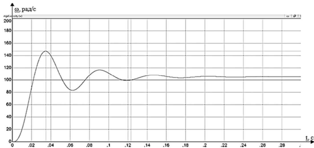
Рис. 9. Переходный процесс при изменении параметра K_{\text{дв}} на –50%
