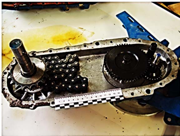
Рис. 1. Редуктор мотокультиватора «Крот» (МК) с двигателем «Robin-Subaru»
