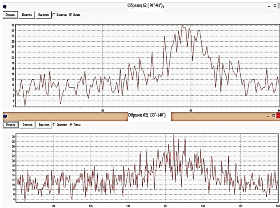
Рис. 1. Фрагмент дифрактограммы образца из сплава 5 ВМЦ, прошедшего насыщение азотом при 550^{\circ}\text{C} в течение 8 часов
