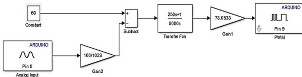
Рис. 3. Модель регулятора, собранная в программной среде Simulink
