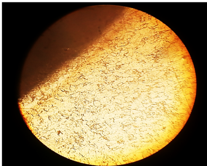
Рис. 6. Микроструктура образца из сплава 5 ВМЦ, прошедшего насыщение при 1000°C 4,5 часа + вакуумный отжиг (x150)
