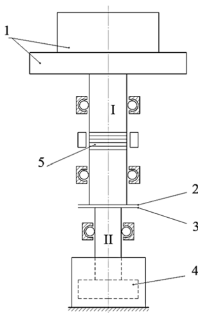
Рис. 1. Кинематическая схема стэнда: 1 – стол с прибором; I – вал стола; II – вал двигателя; 2, 3 – элементы муфты; 4 – ротор двигателя; 5 – ламель токоподвода
