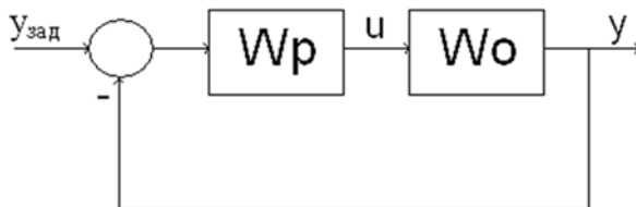
Рис. 1. Упрощенная структурная схема исследуемой системы
