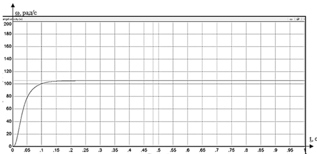
Рис. 10. Переходный процесс при изменении параметра K_{дв} на +50%
