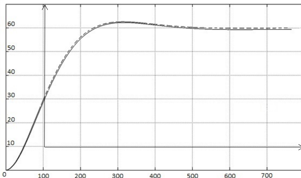
Рис. 5. Переходные характеристики с выхода объекта управления при подаче ступенчатого сигнала равного 60°C
