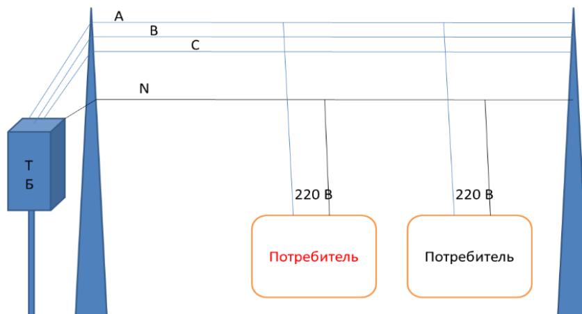
Рис. 1. Схематичное представление преобразования и передачи напряжения потребителю
