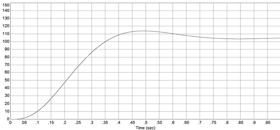
Рис. 5. Переходный процесс по угловой скорости
