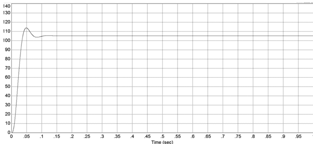
Рис. 4. Переходный процесс для фильтра Баттерворта 3-го порядка
