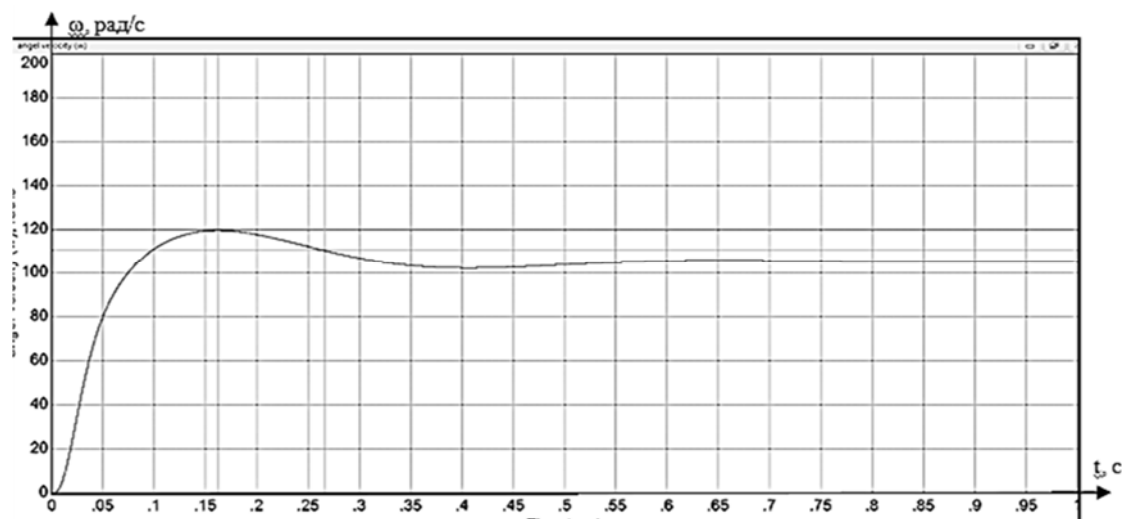
Рис. 8. Переходный процесс при изменении параметра T_M на +50%
