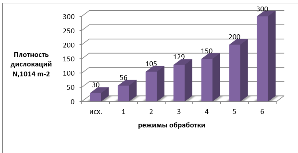
Рис. 4. Диаграмма значений плотности дислокаций сплава 5 ВМЦ. По оси абсцисс введены следующие обозначения: исх. – исходное состояние образца; 1 – насыщение при 550^{\circ}\text{C} – 8 часов; 2 – при 1000^{\circ}\text{C} – 1 час; 3 – при 800^{\circ}\text{C} – 8 часов; 4 – насыщение при 800^{\circ}\text{C} – 10 часов; 5 – при 700^{\circ}\text{C} – 20 часов; 6 – при 700^{\circ}\text{C} – 10 часов
