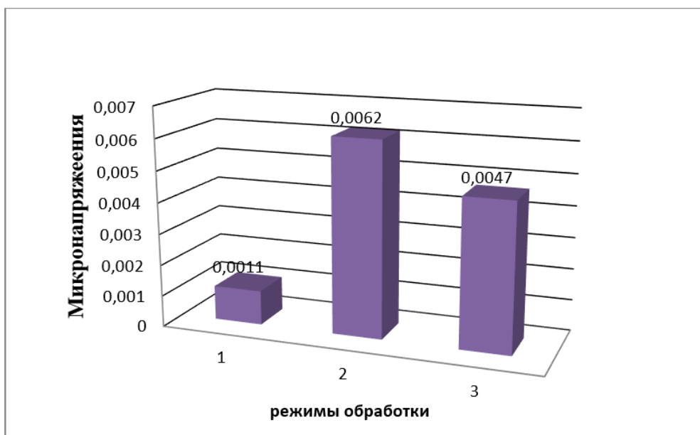
Рис. 3. Диаграмма значений микронапряжений сплава 5 ВМЦ в зависимости от режимов обработки образцов:
