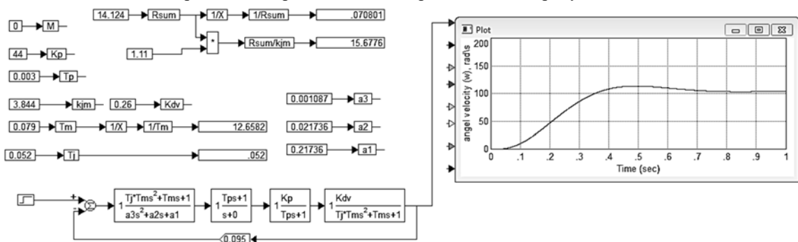
Рис. 3. Модель системы в среде моделирования Vissim
