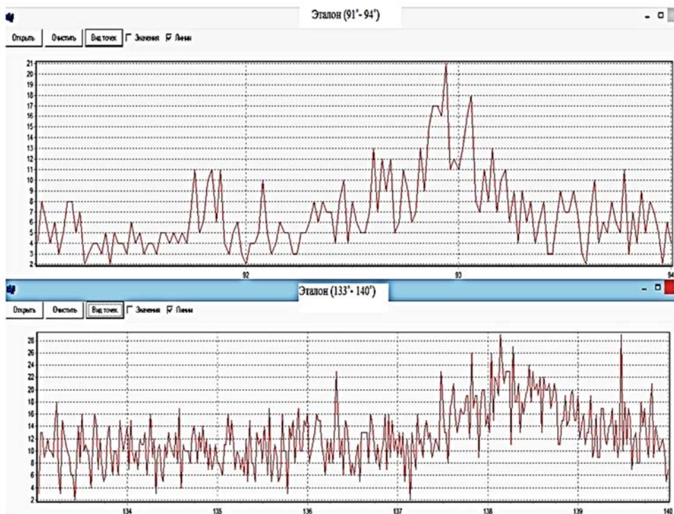
Рис. 2. Фрагмент дифрактограммы эталона
