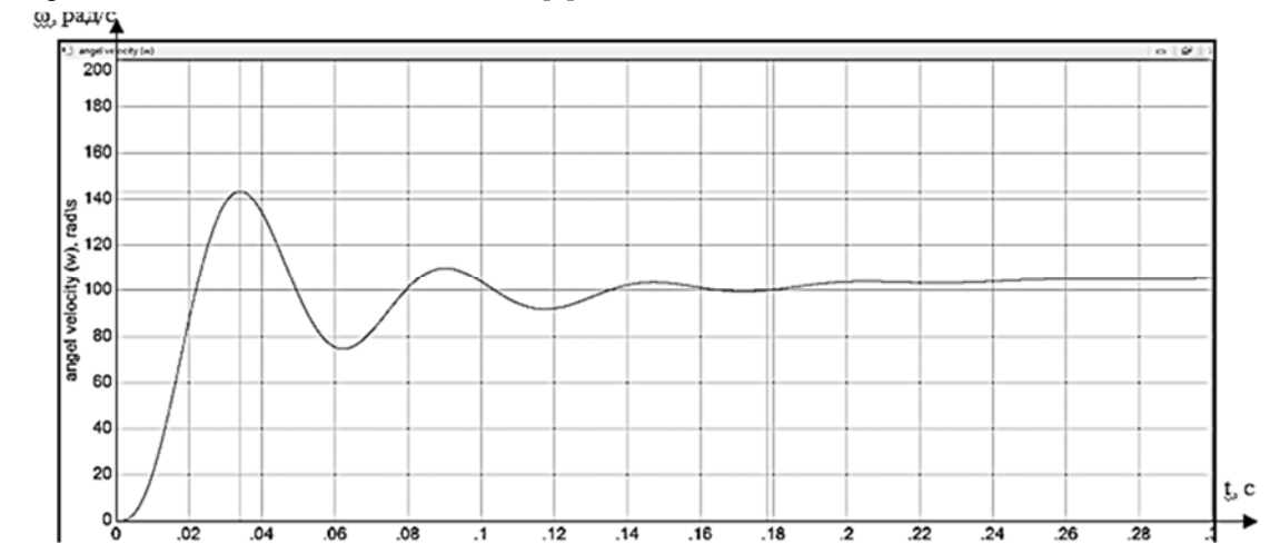
Рис. 7. Переходный процесс при изменении параметра T_M на -50\%
