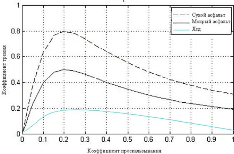
Рис. 1. Псевдостатическая кривая зависимости коэффициента трения от величины проскальзывания колеса
