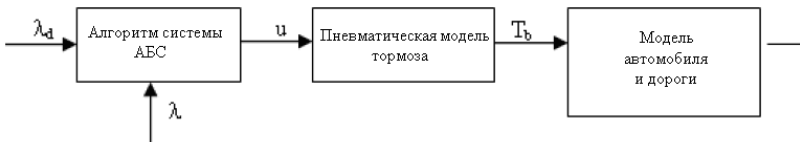
Рис. 2. Функциональная схема управления с помощью системы ABS
