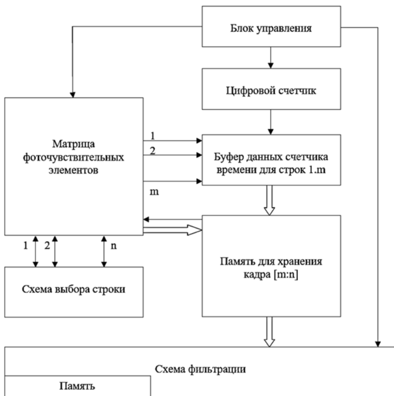
Рис. 1. Структурная схема
