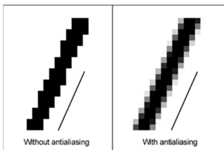
Рис. 1. Алиасинг изображения
