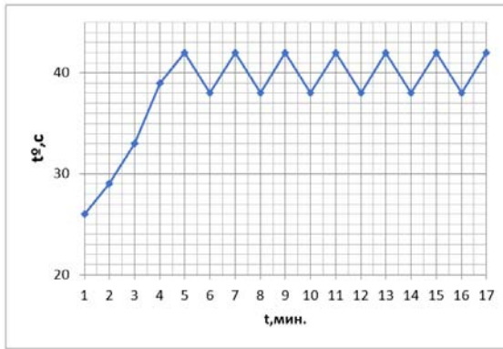
Рис. 2. Экспериментальная зависимость процесса сушки свежееубранного пивоваренного ячменя инфракрасным излучением выделенной длиной волны 1,5–3,0 мкм в осциллирующем режиме при естественном охлаждении продукта при начальном влагосодержании зерен ячменя 17,6 кг/кг, плотности теплового потока 2,3 кВт/м 2 , высоты слоя ячменя на поддоне 10мм при достижении конечных значений влагосодержания ячменя 16,3 кг/кг и температуры 43–44°C
