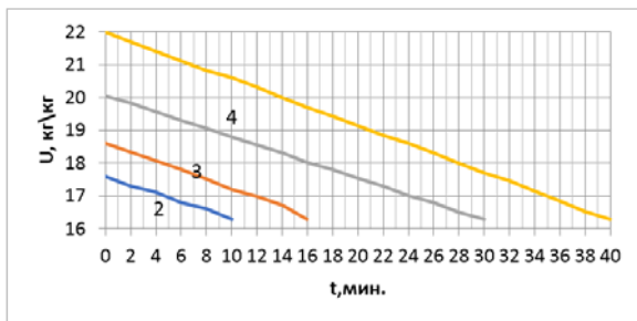
Рис. 3. Экспериментальные зависимости процесса сушки свежесобранного пивоваренного ячменя инфракрасным излучением выделенной длиной волны 1,5–3,0 мкм в осциллирующем режиме при естественном охлаждении продукта в зависимости от начального влагосодержания ячменя 17,6 кг/кг (прямая 1), 18,6 кг/кг (прямая 2), 20,5 кг/кг (прямая 3), 22,0 кг/кг (прямая 4), плотности теплового потока 2,3 кВт/м 2 , высоты слоя ячменя на противне 10 мм при достижении конечных значений влагосодержания ячменя 16,3 кг/кг и температуры 43–44°C
