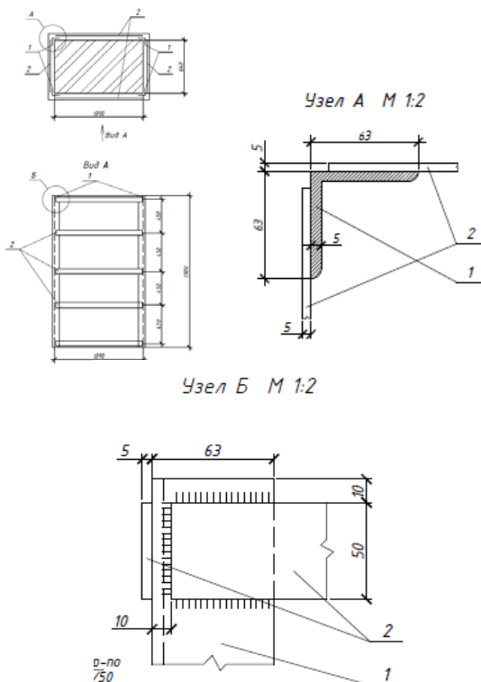
Рис. 6. Схема усиления простенка 1 – уголок 63 х 63 х 5, 2 – полоса 50 х 5
