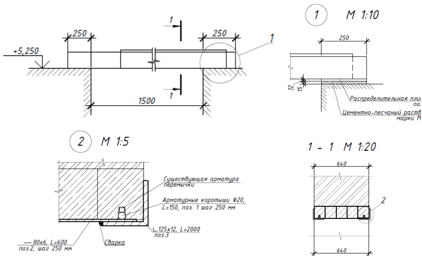
Рис. 5. Усиление перемычки ПР1
