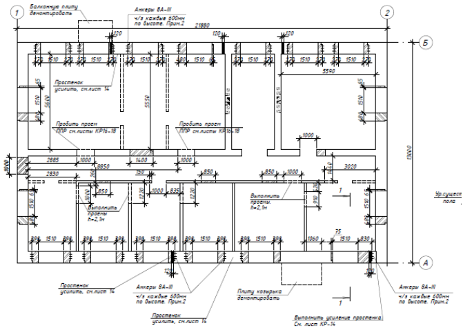
Рис. 3. План демонтажа и устройство проемов 2 этажа
