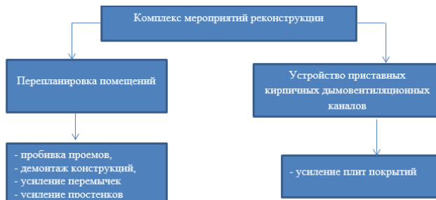
Рис. 1. Комплекс мероприятий при реконструкции жилого дома
