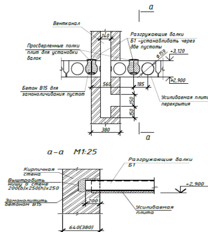
Рис. 7. План разгружающих балок
