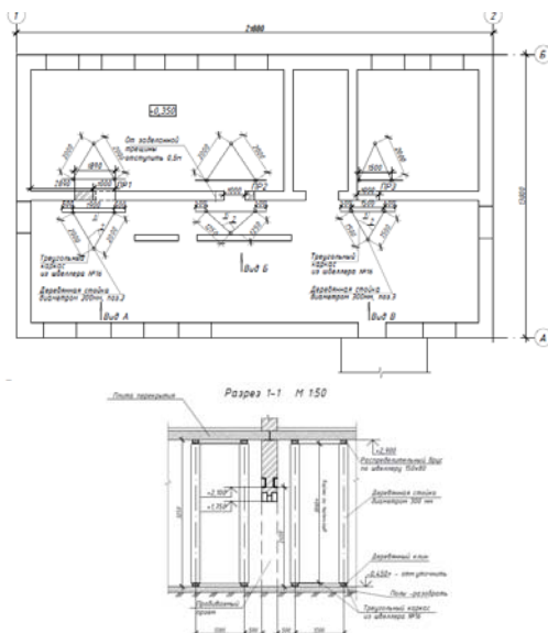
Рис. 4. Схема установки поддерживающих стоек при пробивке проемов в несущих стенах 1-го этажа
