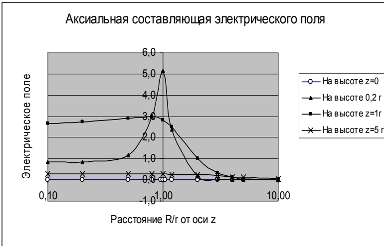
Рис. 10. Аксиальная составляющая электрического поля кольца
