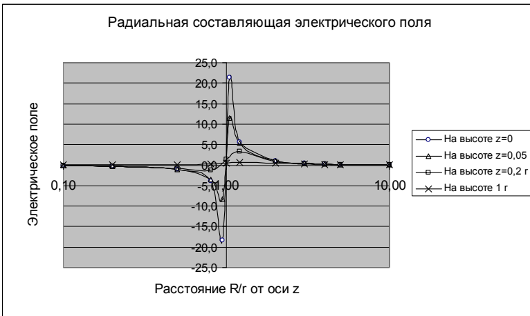
Рис. 9. Радиальная составляющая электрического поля кольца
