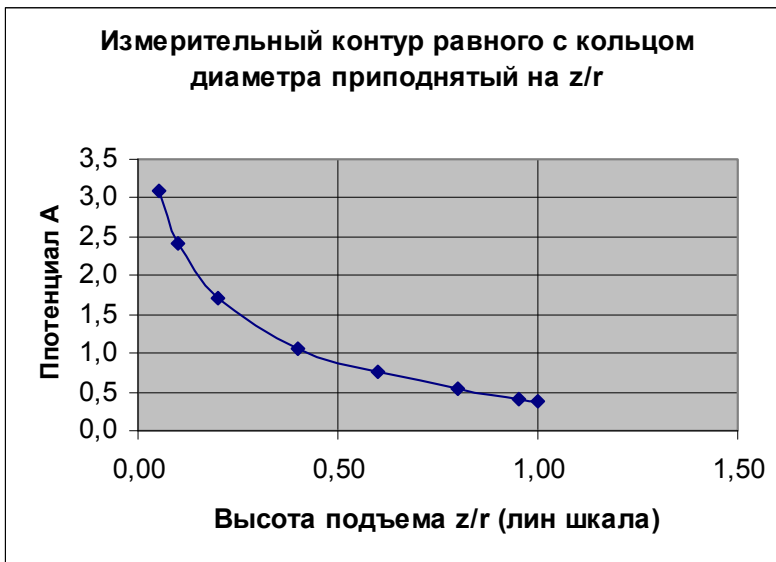
Рис. 19. Графики распределения векторного потенциала кольца с током
